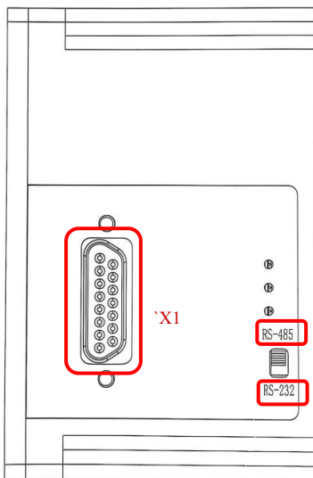
图 1.4 KTP-iR90 型磁悬浮分子泵控制盒面板
