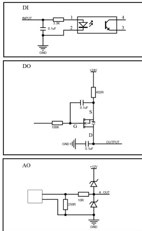
图 1.6 部分接口电路
