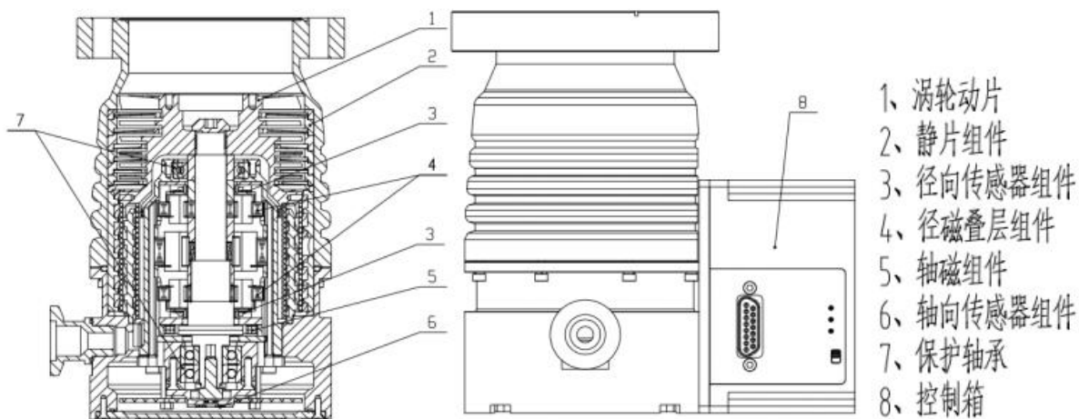
图 1.1 分子泵整机剖面图
