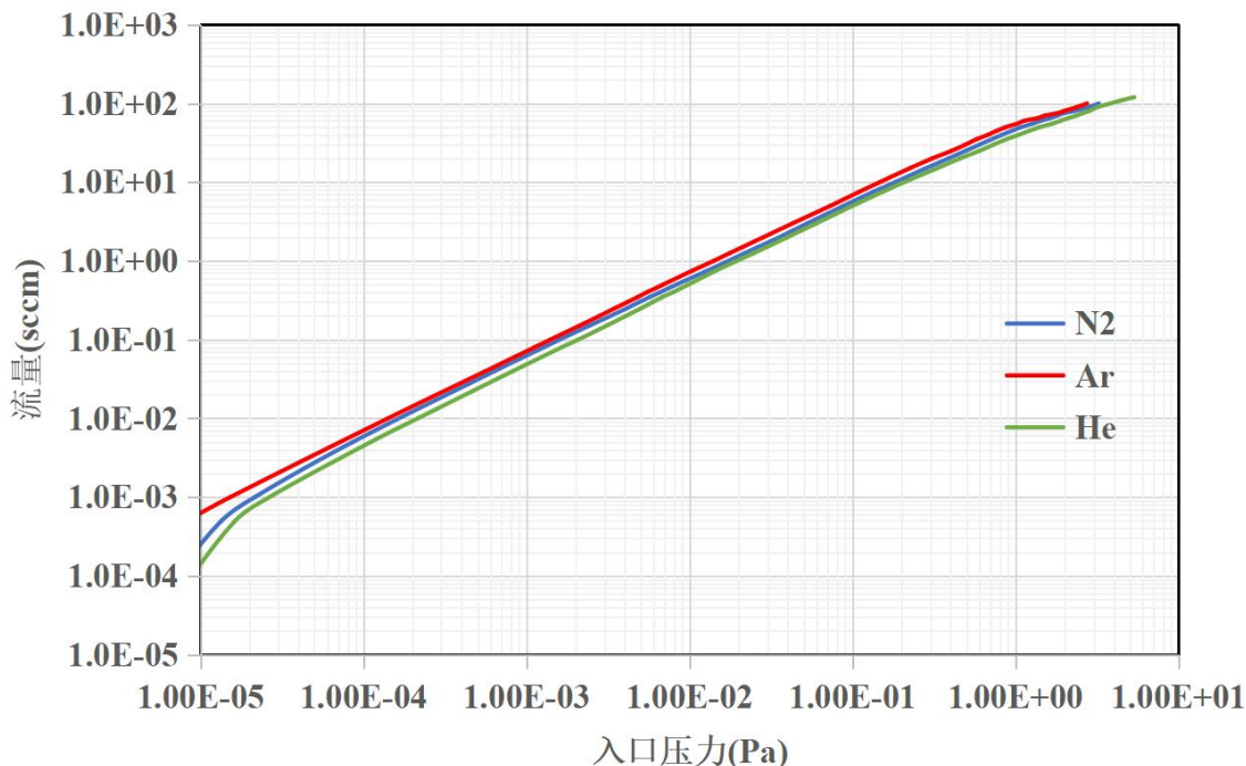
图 2.2 KTP-iR90 流量-压力曲线
