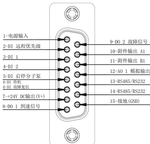
图 1.5 磁悬浮泵接口面板及引脚定义
