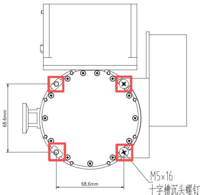
图 3.1 底部安装孔位示意图
