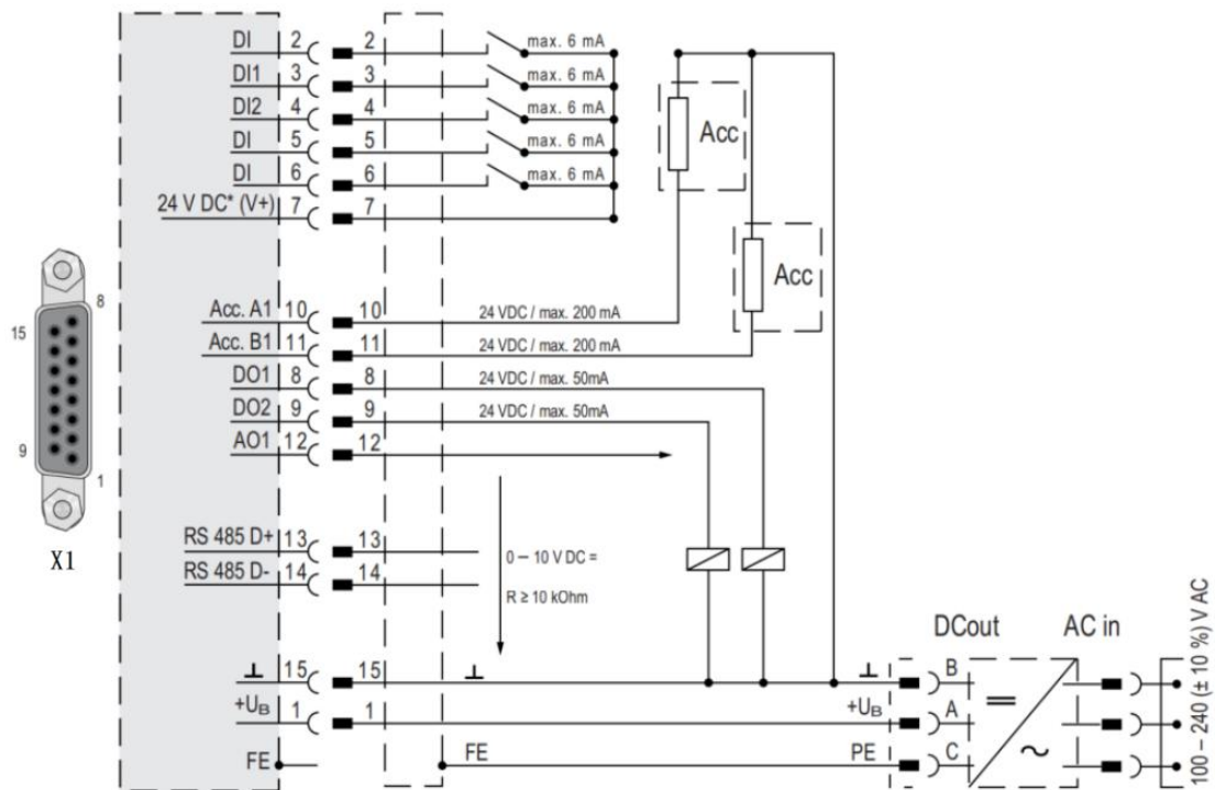
图 1.6 部分接口电路
