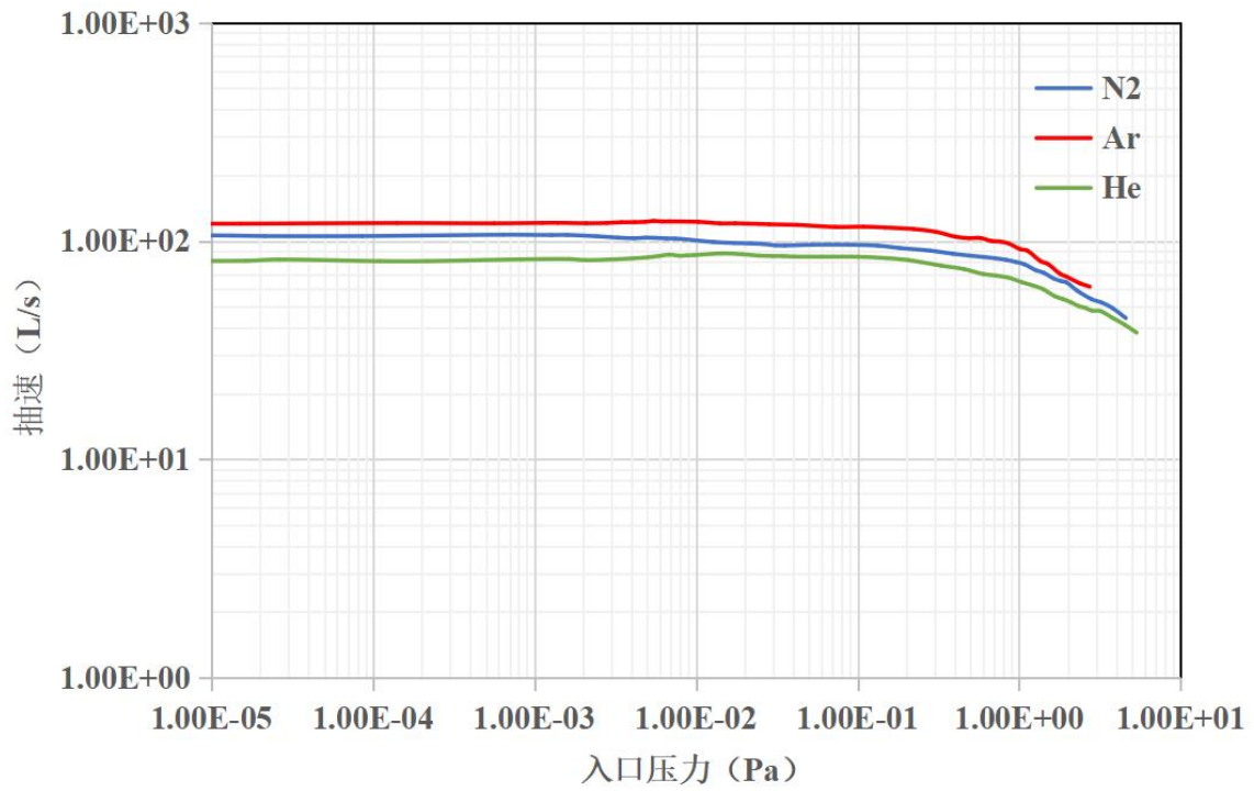
图 2.1 KTP-iR90 抽速曲线
