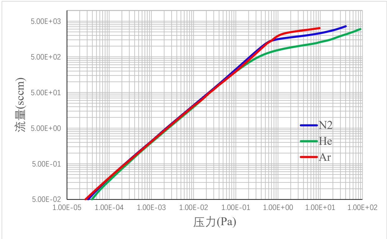
图 2.2 KTP-H3803 系列磁悬浮分子泵额定转速 P-Q 曲线
