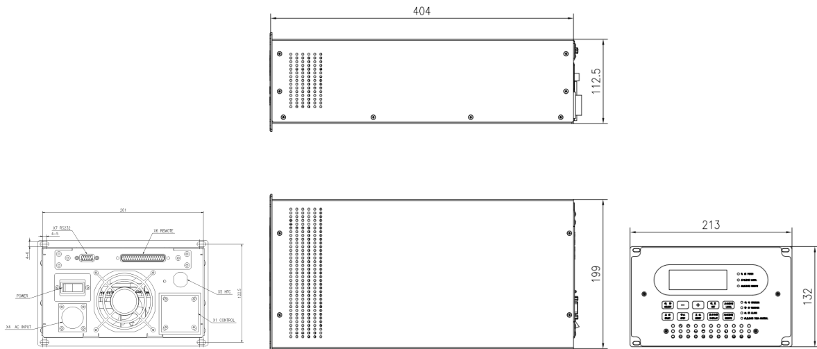
图 1.4 KTC-L0115F(AT)R01 型磁悬浮分子泵控制器
