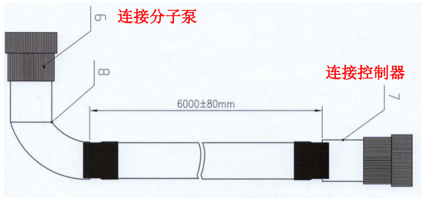
图 1.7 航插线缆及其连接说明
