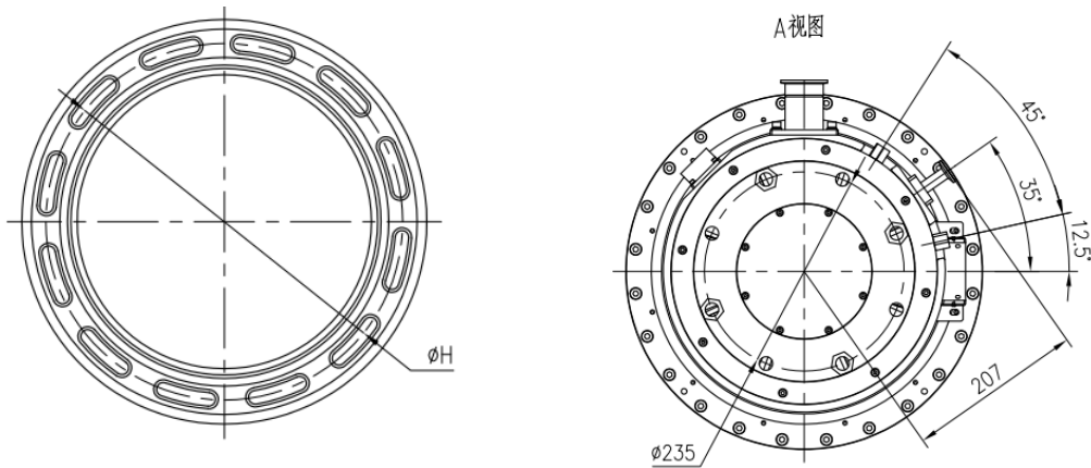
图 1.2 KTP-H4503WCT 型磁悬浮分子泵顶视图及底视图
