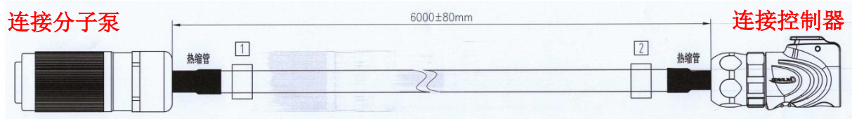
图 1.8 温控线缆及其连接说明
