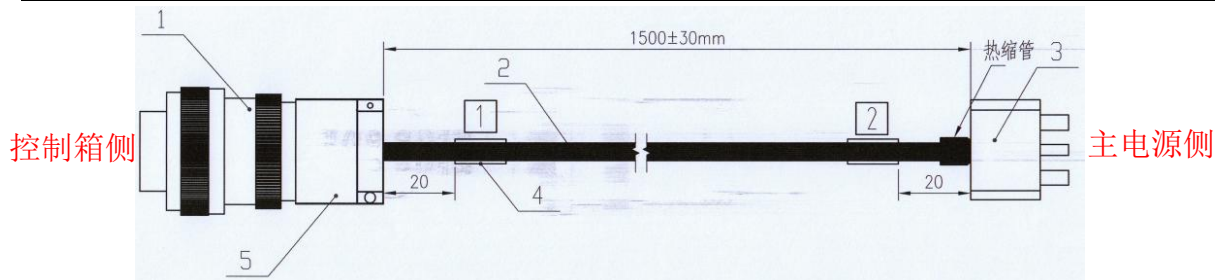
图 1.6 电源线缆及其连接说明
