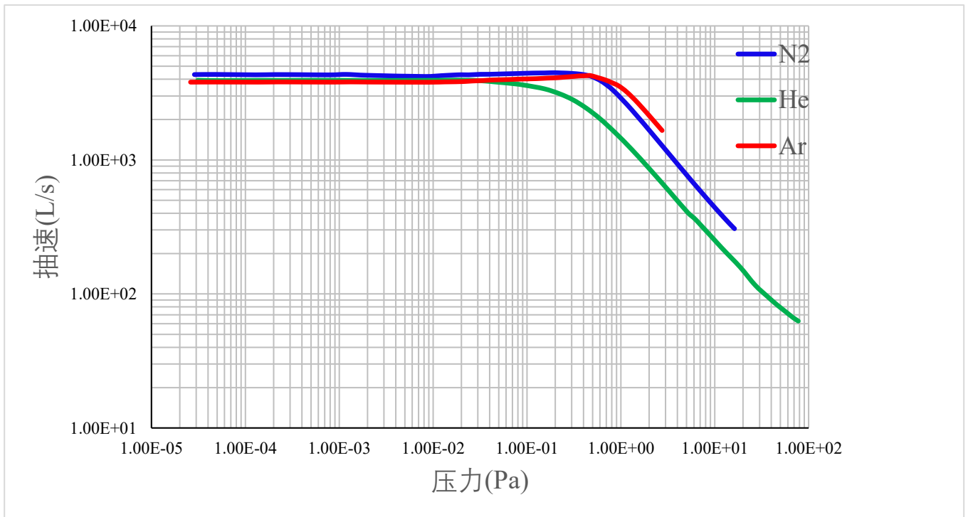
图 2.3 KTP-H4503 系列磁悬浮分子泵额定转速抽速曲线
