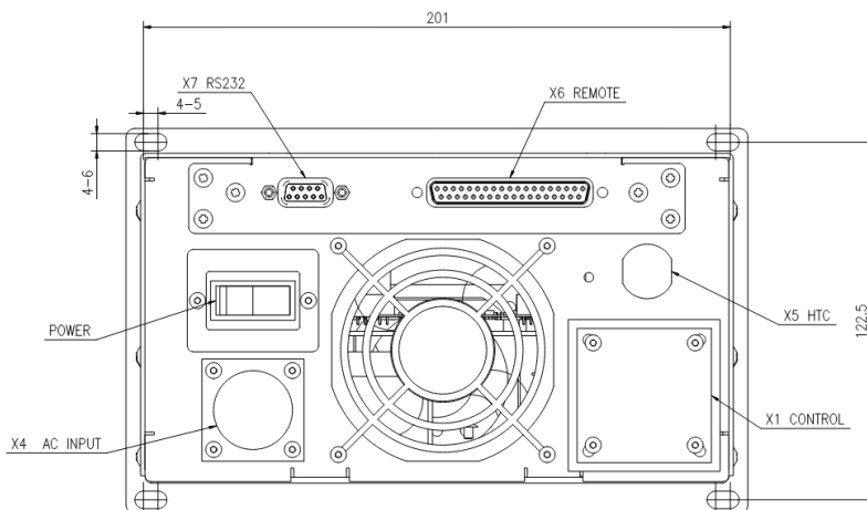
图 1.5 接口面板
