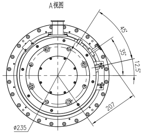
图 1.2 KTP-H4503WCT 型磁悬浮分子泵顶视图及底视图
