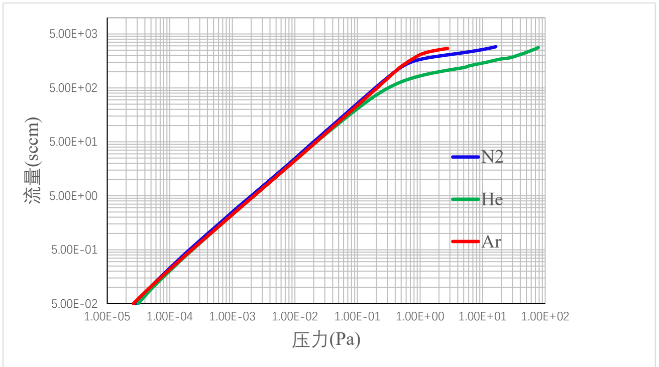
图 2.4 KTP-H4503 系列磁悬浮分子泵额定转速 P-Q 曲线
