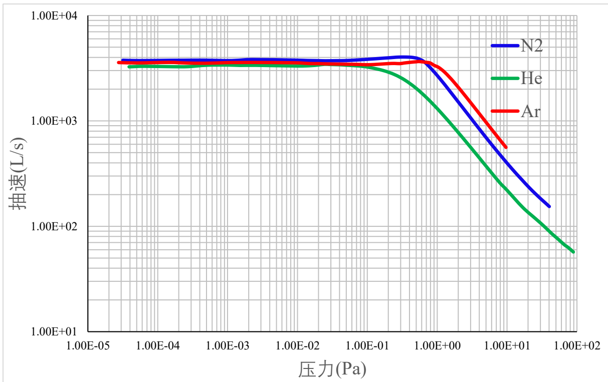
图 2.1 KTP-H3803 系列磁悬浮分子泵额定转速抽速曲线
