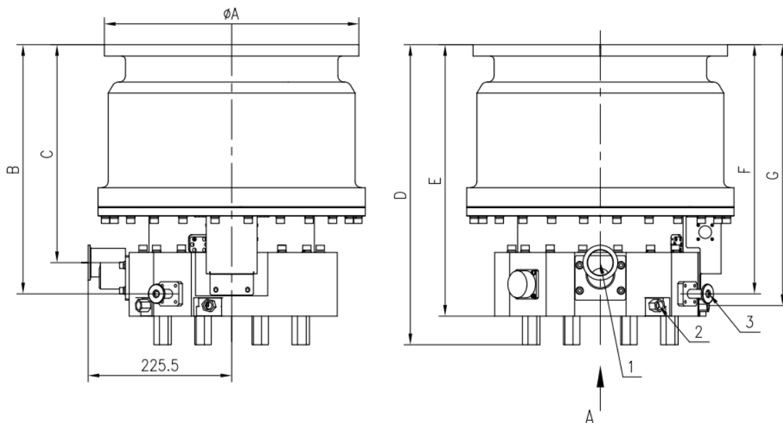
图 1.3 KTP-H4503 系列磁悬浮分子泵顶视图与主要外形尺寸图
